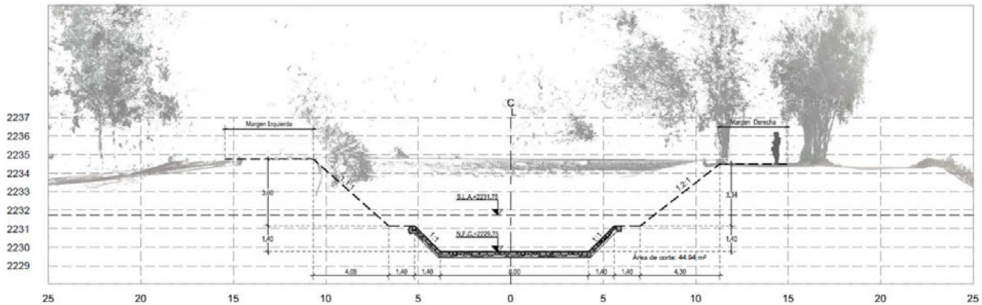
Estación 6+340.00 - Detalle de cortes de terreno
