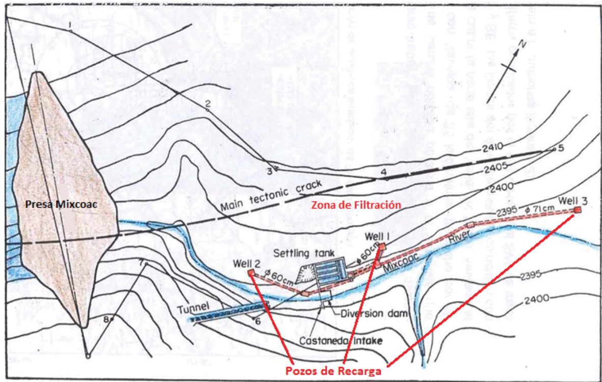
Pozos de infiltración en las márgenes del Río Mixcoac
